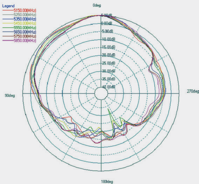
5G (PHI=0)
