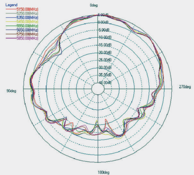
5G (PHI=90)
